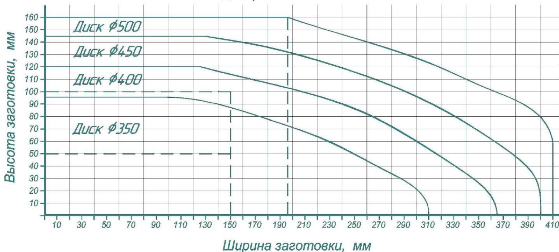
Диаграмма пиления
